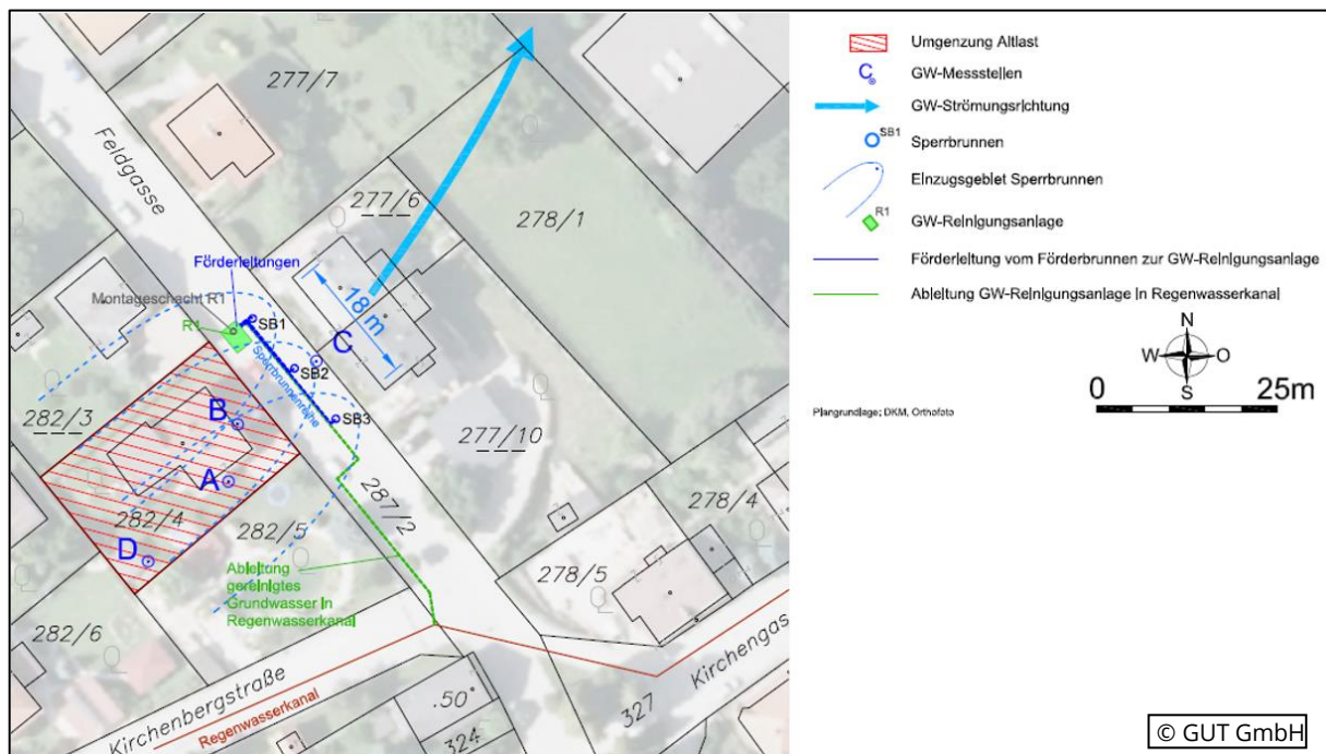
Abbildung 3: Lage der Sperrbrunnen, der Sicherungsanlage und der Grundwassermessstellen im Bereich des Standortes
