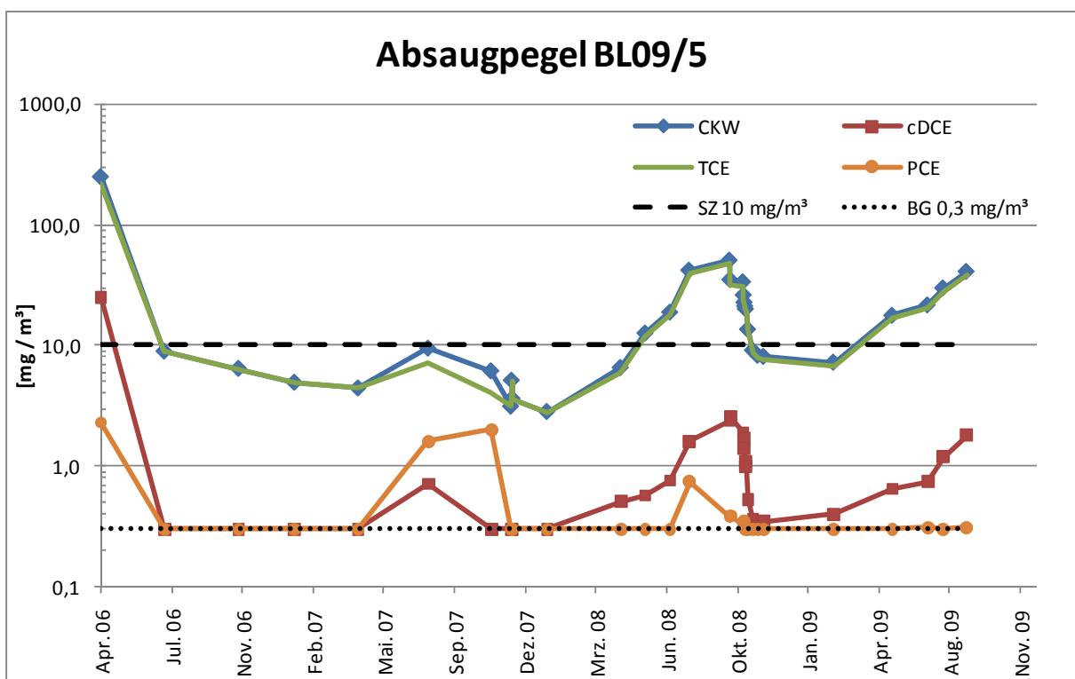
Abb.5: Konzentrationsverlauf ausgewählter CKW am Absaugpegel BL09/5
