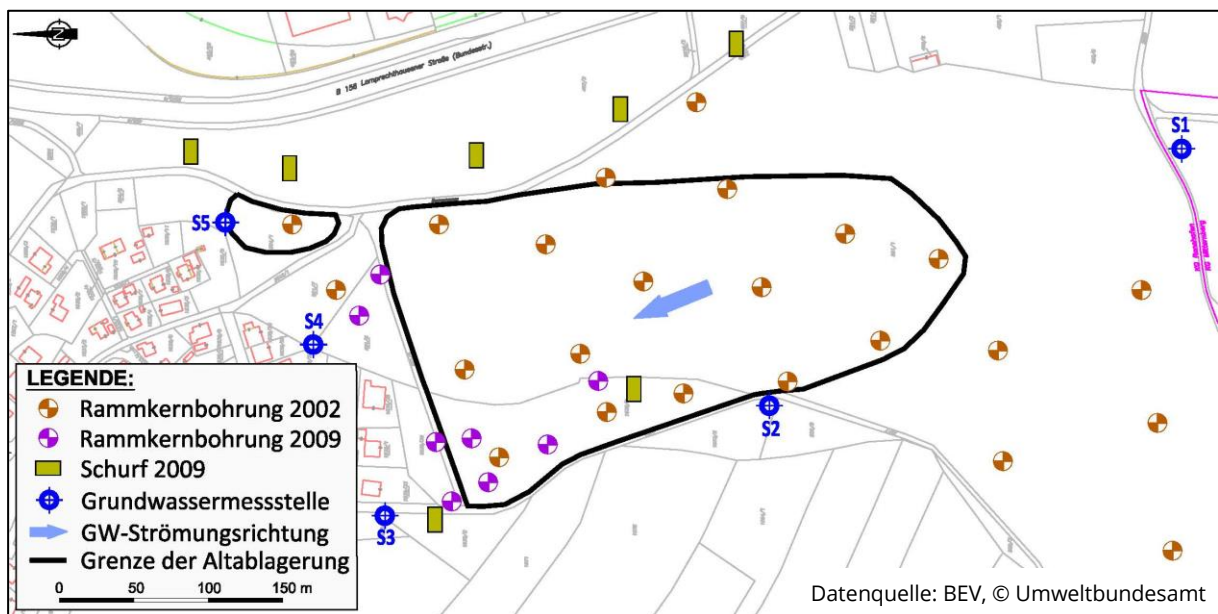
Abb. 5: Lageplan der Untergrundaufschlüsse und Grundwassermessstellen
