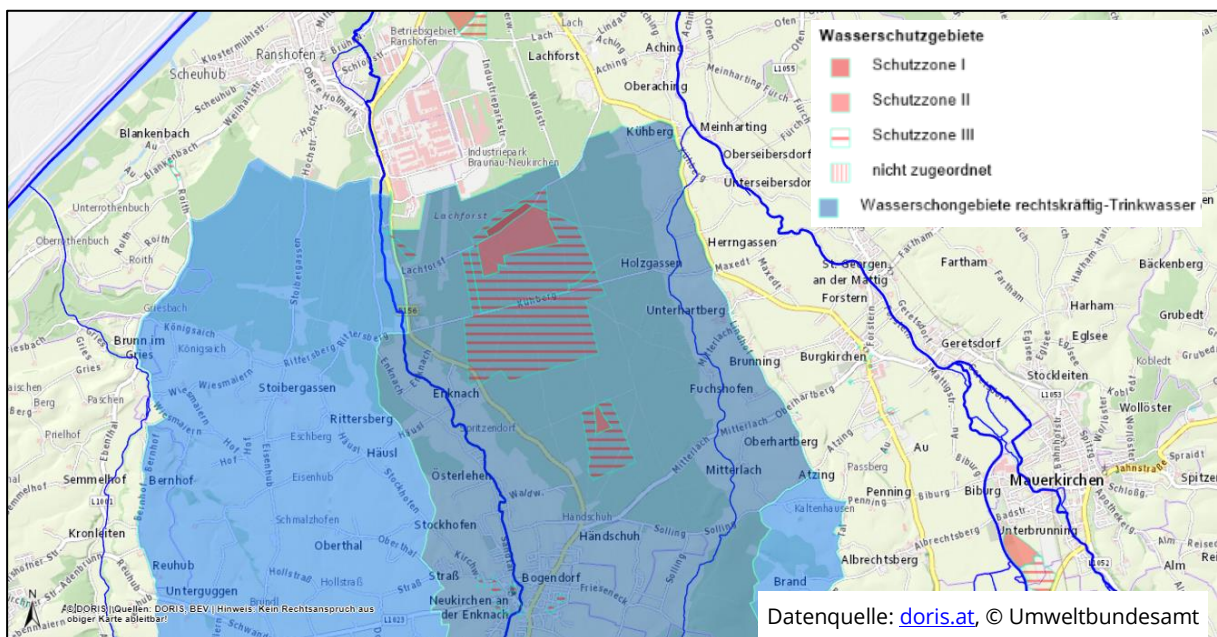
Abb. 4: ausgewiesene Grundwasserschutzzonen
